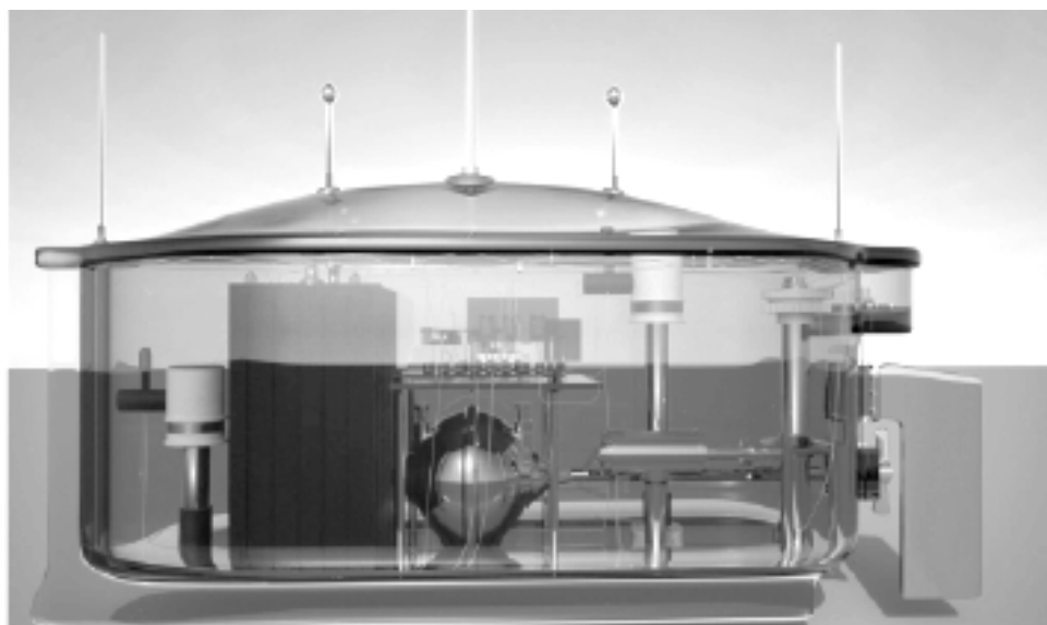
3D kompjuterski model Teslinog teledirigovanog brodića
